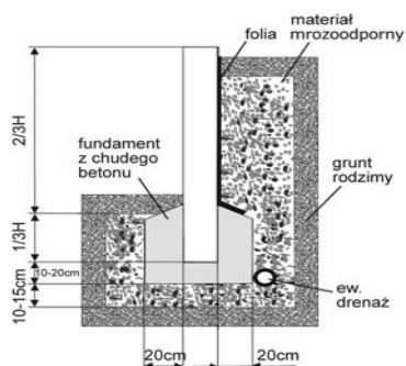
Rys. 1. Kształt palisady betonowej chodnikowej
